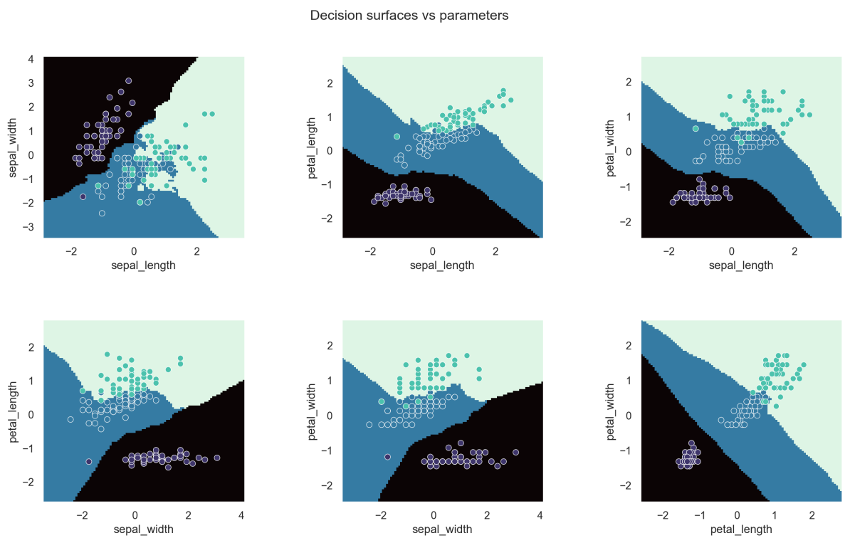
FIGURE 2 – Résultats de l'apprentissage de l'algorithme KNN sur le jeu de données de l'iris. Les régions de décisions du classificateur sont superposées aux valeurs vraies des espèces d'iris.
