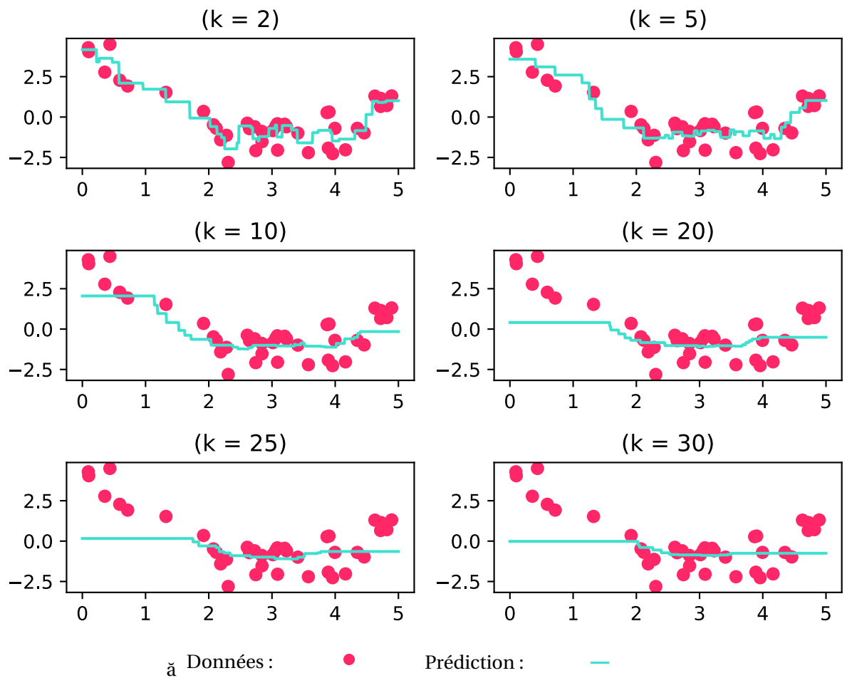
FIGURE 4 – Illustration de l'influence du nombre de voisins k sur une régression de modèle non linéaire dans le cadre de l'algorithme KNN
