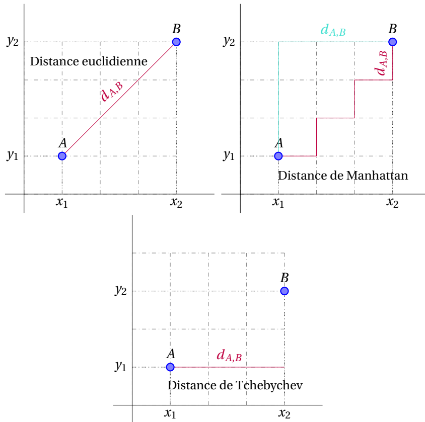
FIGURE 3 – Illustration des différentes distances dans le plan
