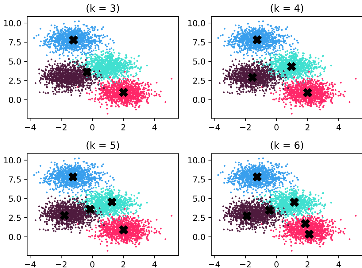
FIGURE 6 – Illustration des conséquences du choix du paramètre k dans k -moyennes. Sur cet exemple, seules quatre classes existent dans les données. k varie entre 3 et 6. Les barycentres sont représentés par des croix noires.
