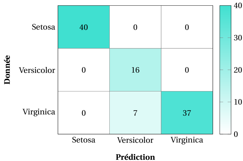
FIGURE 5 – Matrice de confusion dans le cadre de la classification des variétés d'Iris : Setosa, Versicolor et Virginica. Les paramètres d'entrées sont les largeurs et longueurs des pétales et sépales. La prédiction est correcte dans plus de 90% des cas comme le montre la matrice de confusion.
